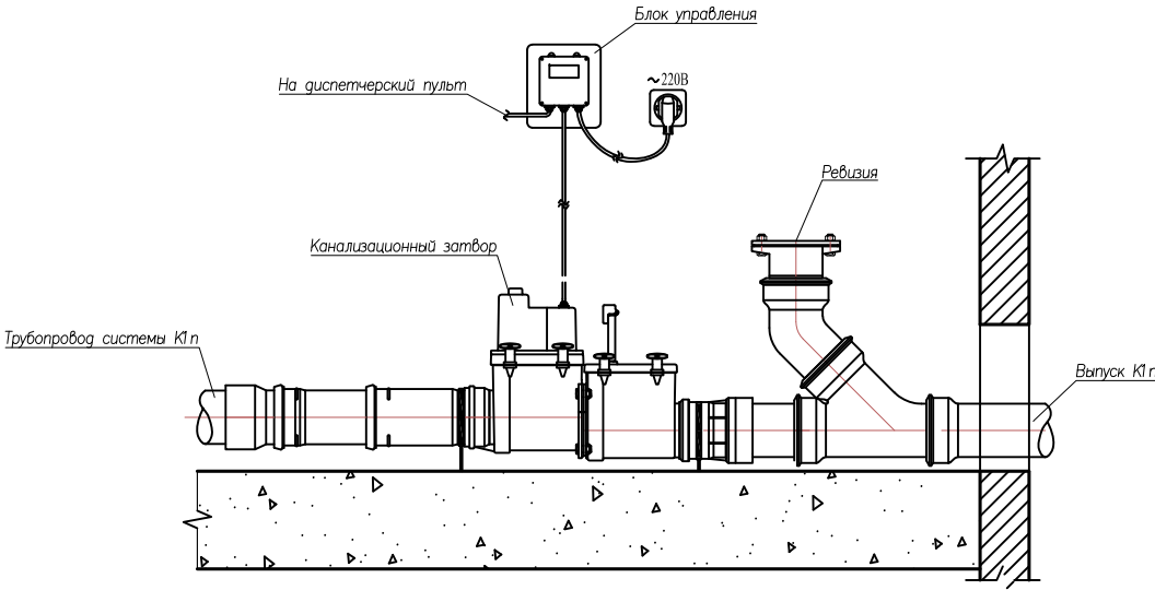
Узел монтажа канализационного затвора
