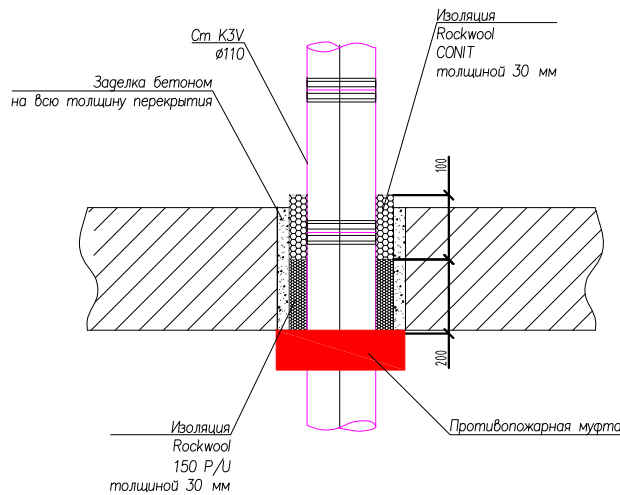
Узел прохода стояков канализации через перекрытия
