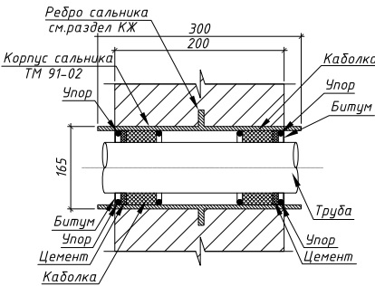
Узел прохода трубопроводов через наружную стену (серия 5.900-20)
