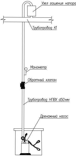
Узел монтажа дренажного насоса
