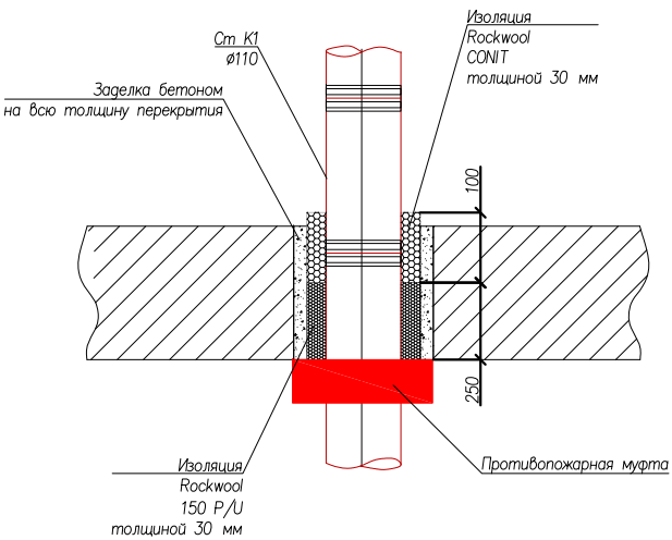
Узел прохода стояков канализации через перекрытия
